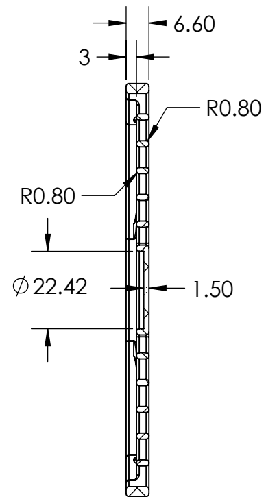
SECTION A-A
